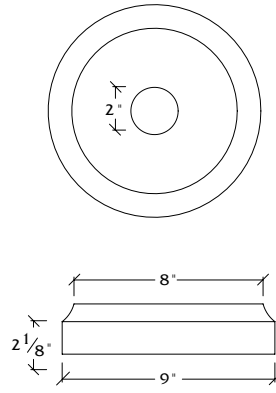
C-2 Collar
