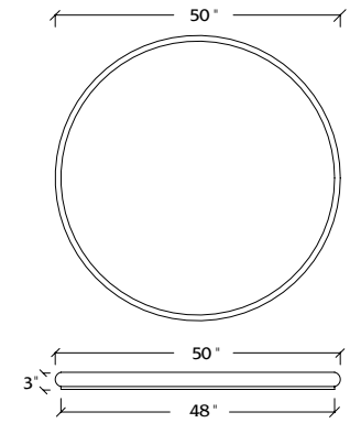
RD-T Table Top
