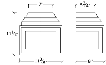
Corbel Plinth
