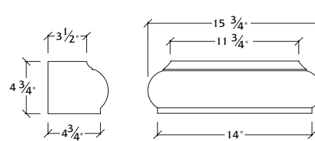
P-16 Plinth
