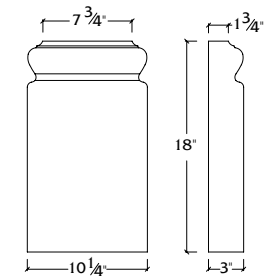
P-10 Plinth
