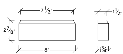
P-8 Plinth
